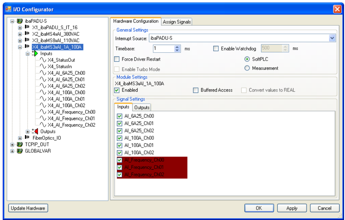
Рис. 14: Входы ibaMS3xAI-1A/100A
