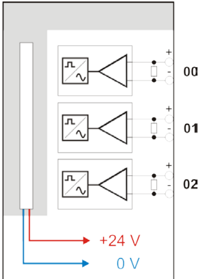
Рис. 4: Схема соединений ibaMS3xAI-1A и ibaMS3xAI-5A
