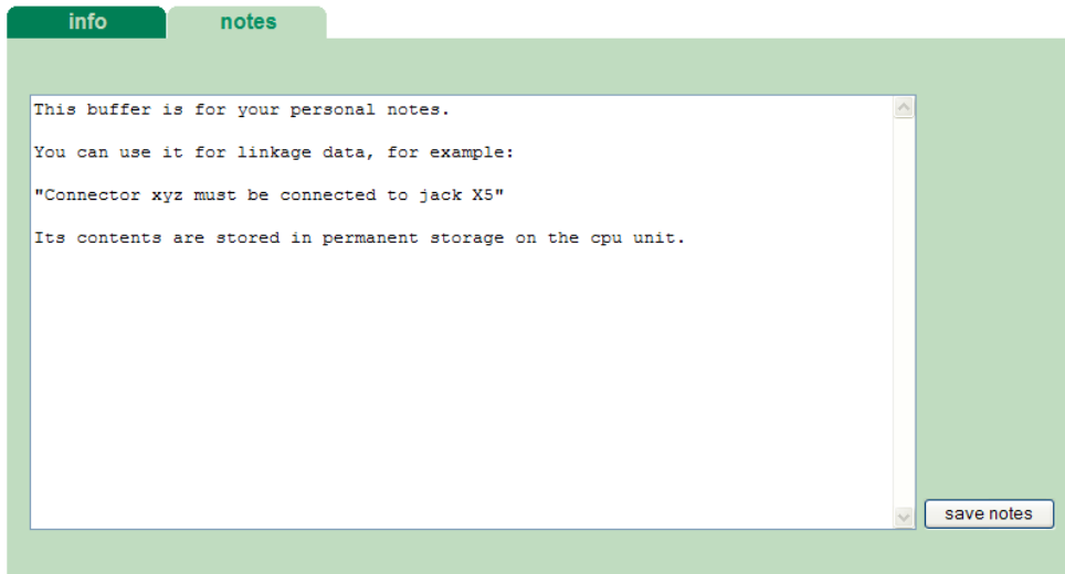
Рис. 9: Вкладка „notes“
