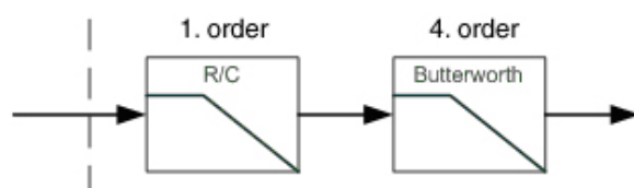
Рис. 3: Секции фильтра
