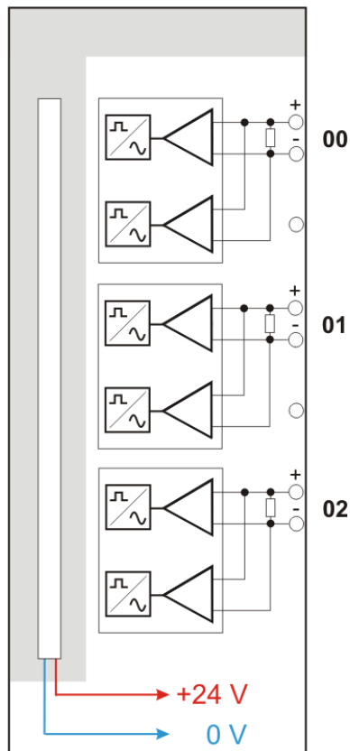
Рис. 5: Схема соединений ibaMS3xAI-1A/100A
