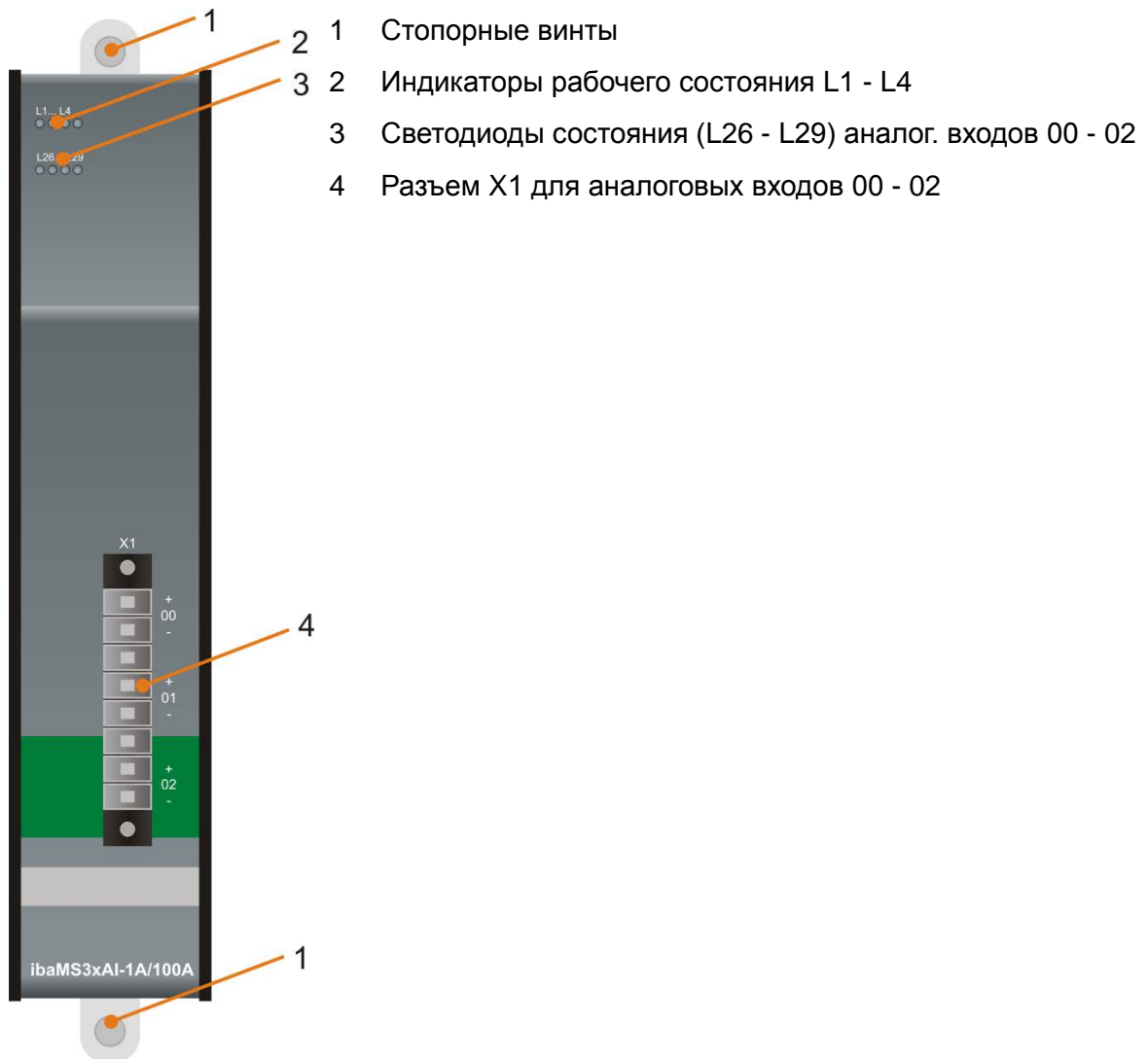
Рис. 1: Вид спереди
